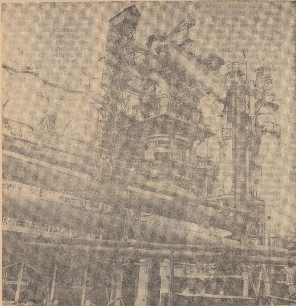
Noul furnal de 700 mc intrat recent în funcțiune la Combinatul metalurgic din Resița. Acest furnal produce anual o cantitate de fontă de peste două ori mai mare decît întreaga producție din anul 1938.
