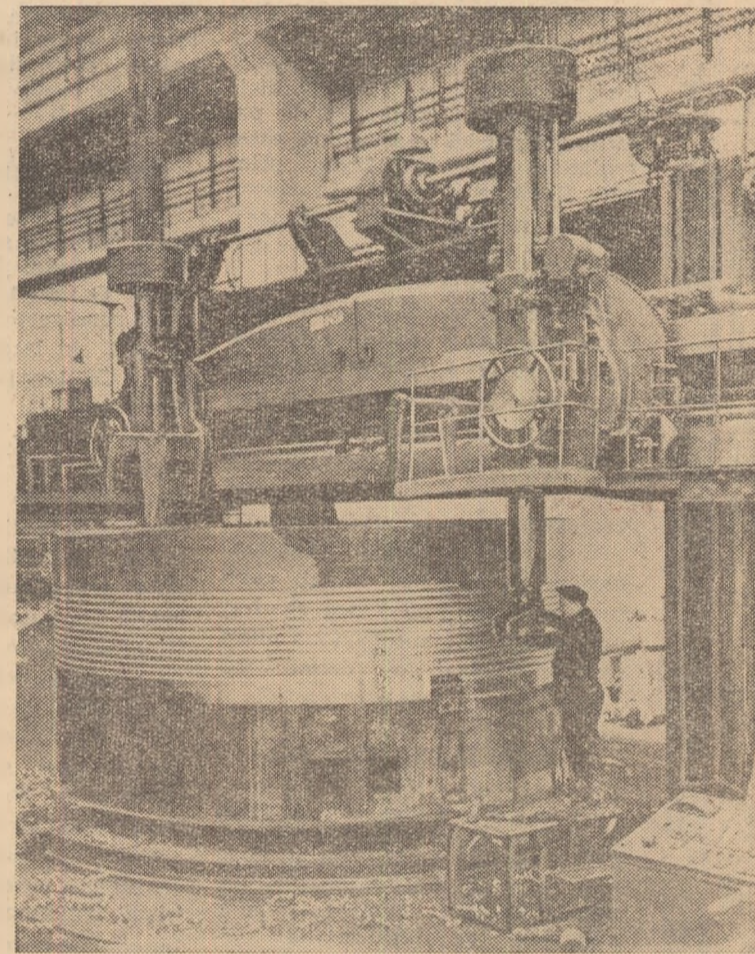
Strungarul G. Lazariov, autorul perfecționării unui strung-carusel, lucrează la acest strung uriaș al uzinei constructoare de mașini „I. V. Stalin” din Novo-Kramatorsk.
