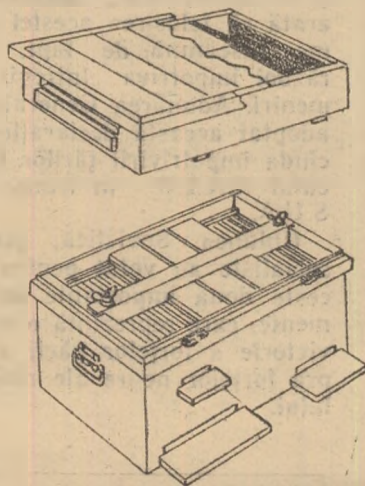
VEDEREA GENERALĂ A STUPULUI ORIZONTAL STAS 4.170-53
