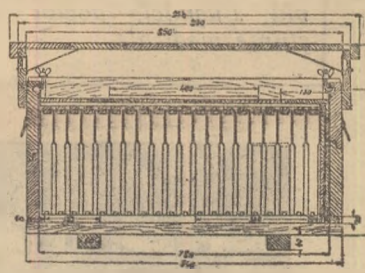
SECȚIUNE PARALELĂ CU URDINIȘUL
