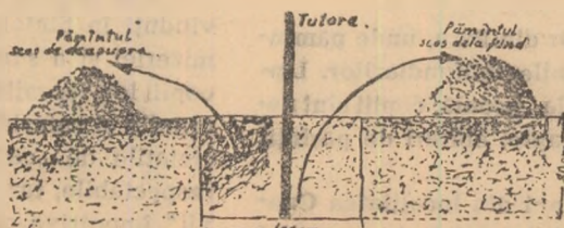
Fig. nr. 4 Groapă pentru plantat pomii
