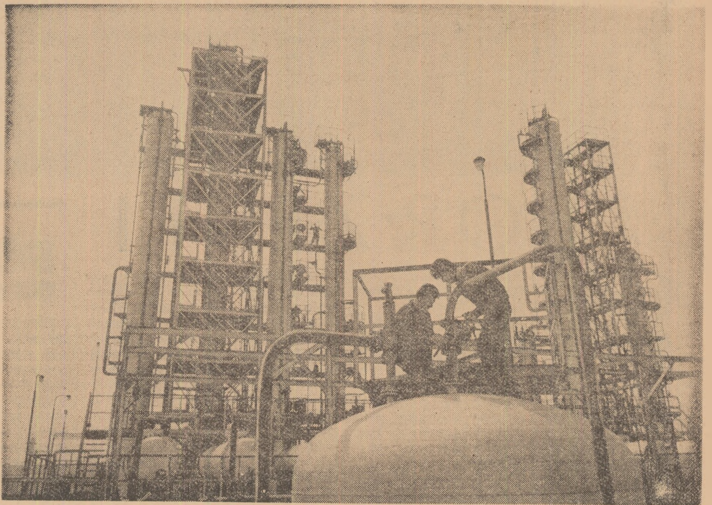
Din noul peisaj industrial al patriei: Combinatul de cauciuc sintetic de la Onești (vedere parțială).
