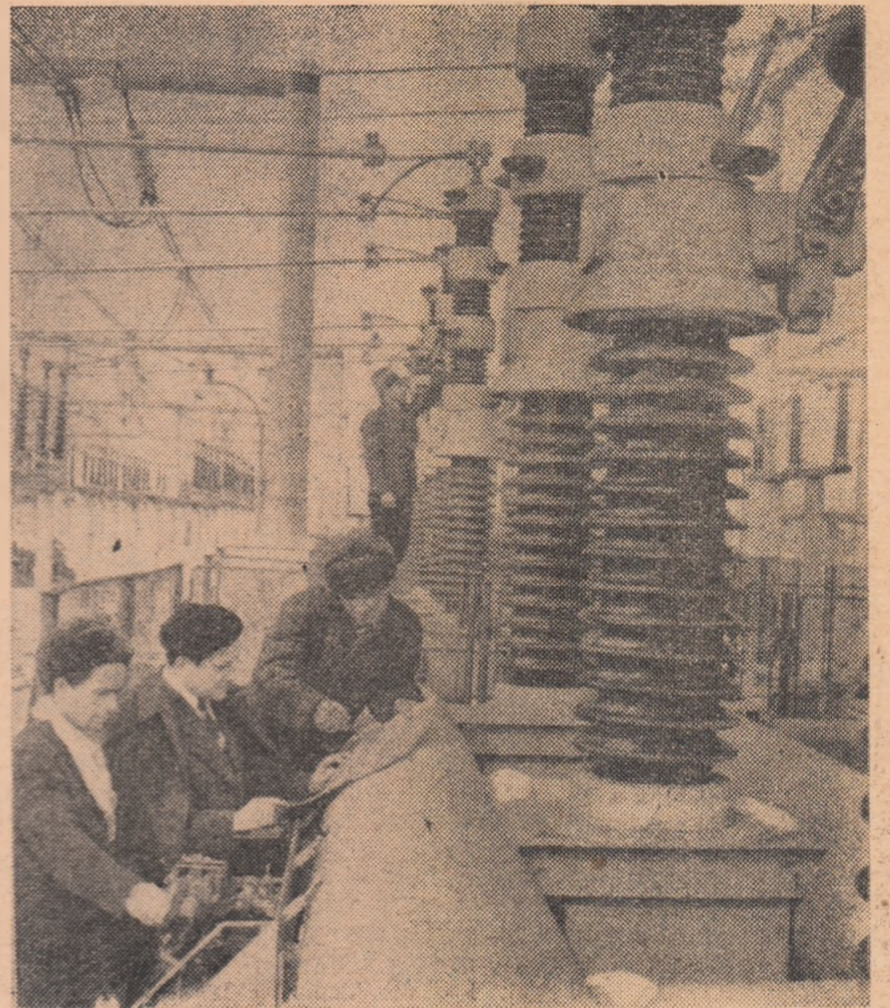
Un aspect de la staţia de 110 000 volţi a centralei.
