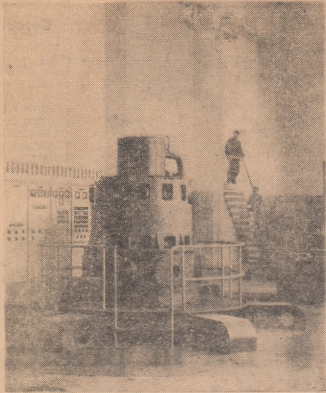
Hidrocentrala Roznov II — sala mașinilor și tablourilor de comandă
