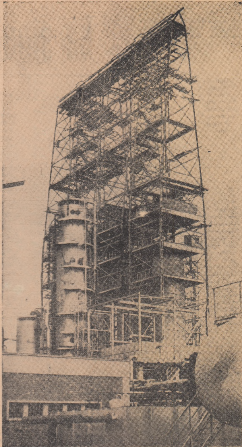
Din noul piesaj industrial: Instalația de coacere întârziată de la rafinăria Brazi.
