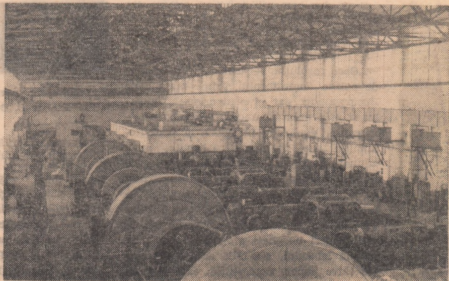
Hala de compresie a secției de amoniac de la Combinatul de îngrășăminte azotoase din Piatra Neamț.
