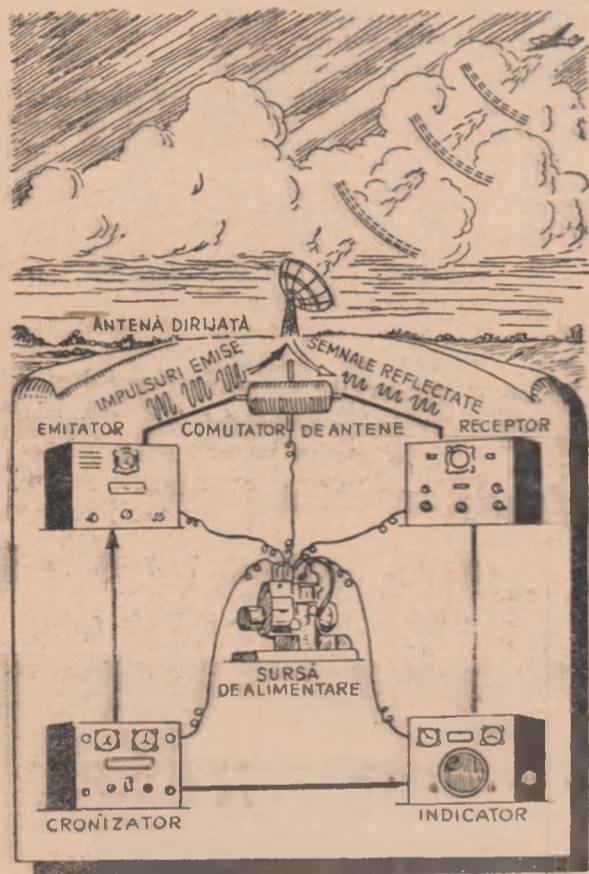
Schema unei stații de radiolocație.
