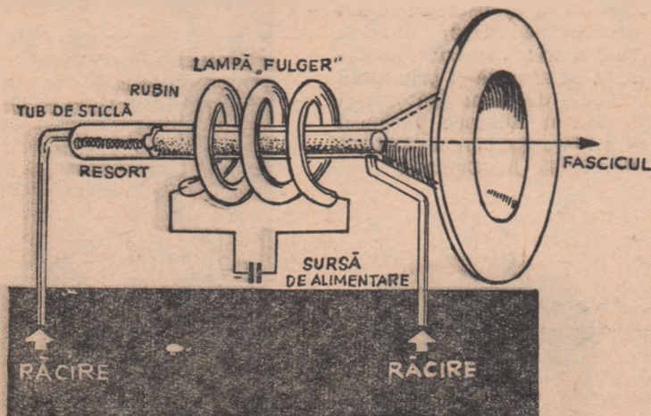
CONSTRUCȚIA LASERULUI
