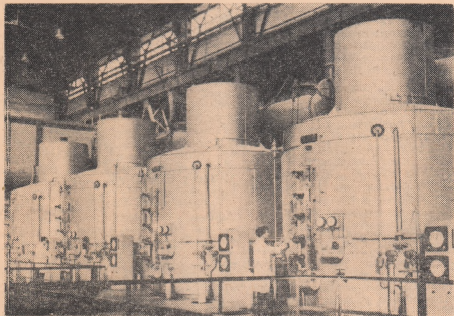
La fabrica de zahăr din Bucecea, procesul de producție este mecanizat și automatizat. În fotografie, operatorul Cheorghe Mindru.
