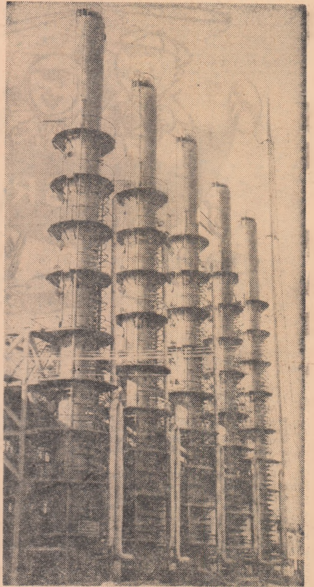
Coloanele de sinteză ale fabricii de acid azotic, din cadrul Combinatului de prelucrare complexă a gazelor — Craiova
