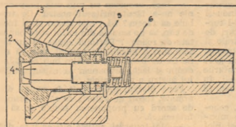
1. Manșon cu con; 2. Bucșă extensibilă; 3. Placa cu filet; 4. Tampon (dorn) reglabil; 5. Pulițe crestate; 6. Resortul.
