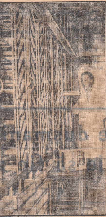
În anul 1953 s-a experimentat la gospodăria agricolă de stat din Aradului No. „Incubatorul industrial B”, cu o capacitate de 64.000 de ouă. Acest incubator a fost conceput de inginerul Ion Dănculescu — laureat al Premiului de stat — și este unul dintre cele mai bune incubatoare din Europa.
