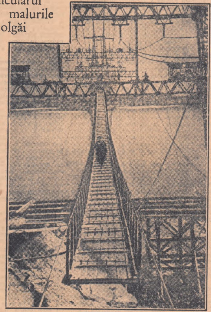
Puntea suspendată de funicularul ce traversează Volga în apropierea Stalingradului.
