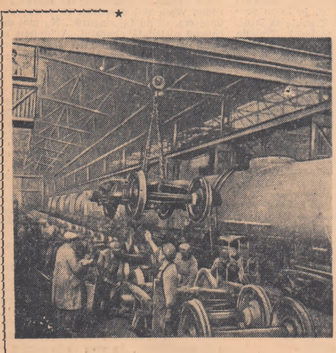
Uzinele „23 August” din București, stăpînite și conduse de către oamenii muncii, și-au lărgit considerabil producția. În fotografie: la secția vagoane se montează acum în serie boghurile pentru vagoane-clsternă C.F.R. de 50 tone. (Foto: AGERPRES)
