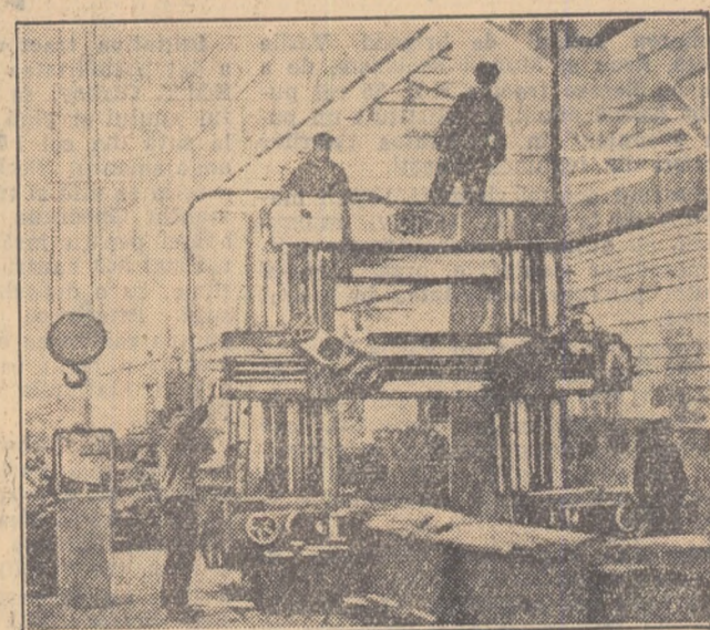
Un aspect de la montarea unei mari instalații la fabrica de automobile din R. P. Chineză.
