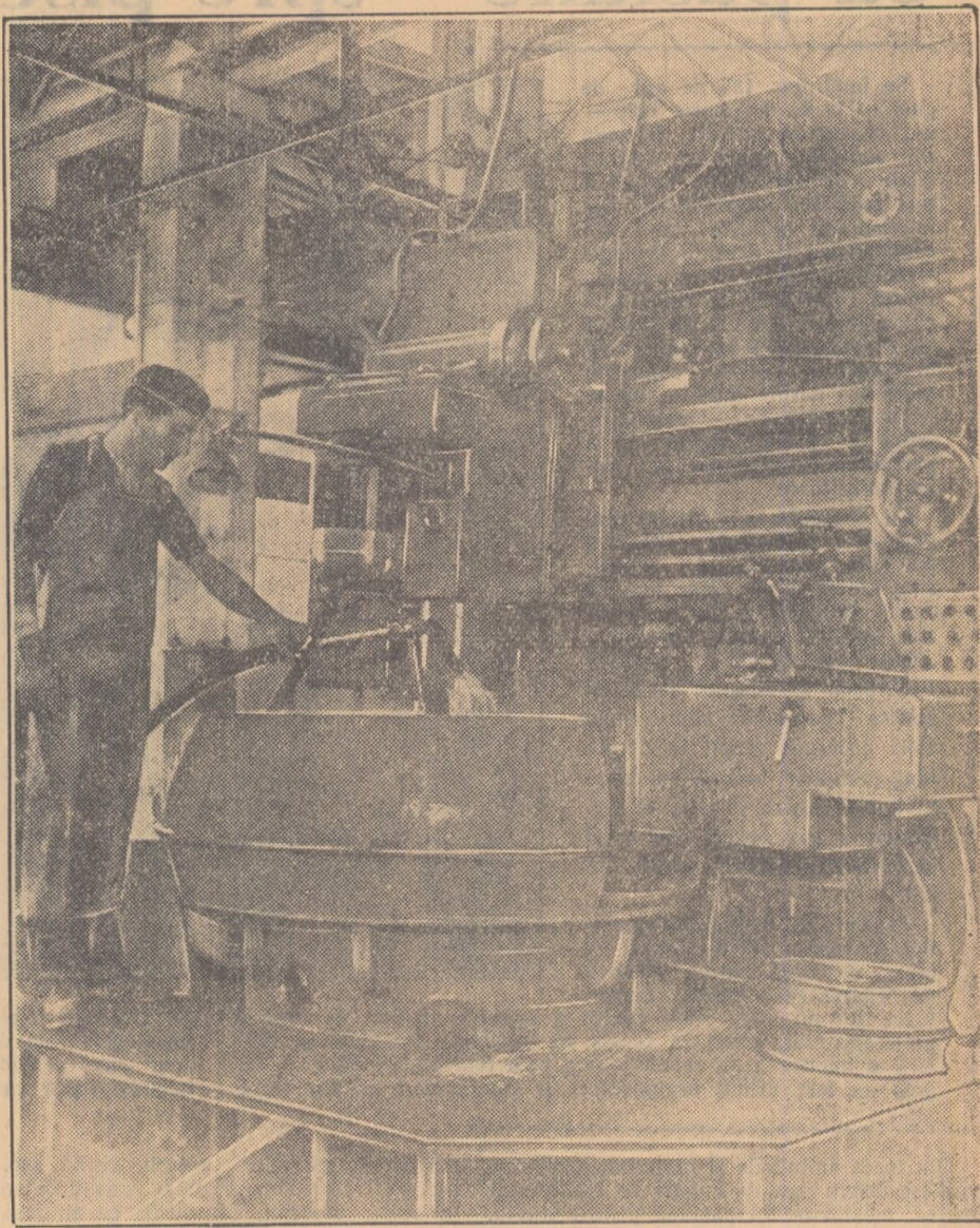
La această mașină modernă sovietică de rectificat căile de rulare ale rulmenților de mare dimensiune, lucrează utemistul Ion Bolat. El este unul dintre fruntașii fabricii de rulmenți din Moldova care în cinstea Congresului partidului realizează zilnic cite două norme.
