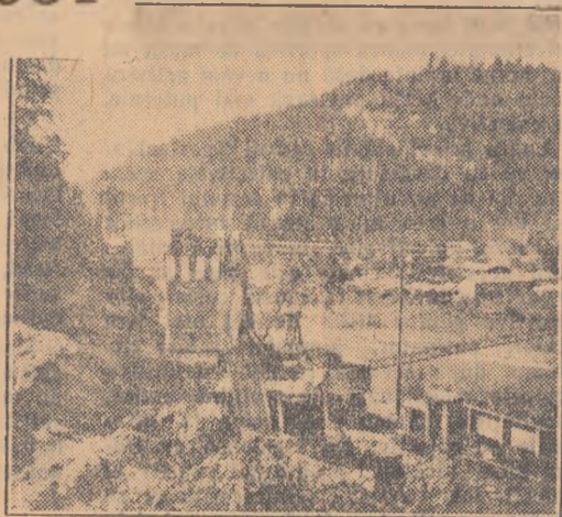
BICAȘ. — Cupele escavatoarelor muscă pentru itilia oară din mărurile Bistriței.
