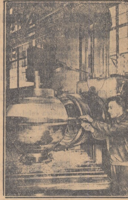
Meșterul comunist Eremia Pitș, de la sectorul mașini uneltelor la uzinile „Steagul roșu“ din Orașul Stalin, se mîndrește cu mulți muncitori pe care i-a crescut. În fotografie: utemistul Eremia Kocșis, calificat recent, executînd strîngerea șterei pentru capul buteliei de apă de 400 atmosfere. În primele zile ale celui de-al II-lea cîncinal el a depășit norma cu 50 la sută. Foto: EUGEN CSIKOS
