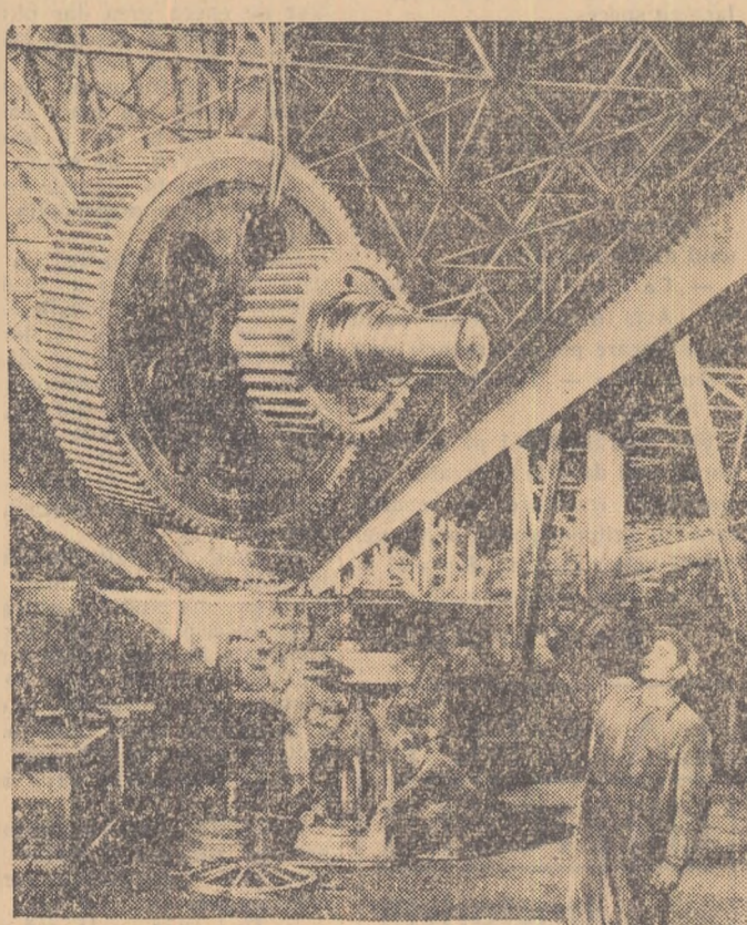
Laminorul de la Roman. În secția reviziei și premonajii tovarășul Simoș Vasile cu echipa sa pregătește roata dințată cu o greutate de 3.500 kilograme, pentru montajul cablului de la laminor.
