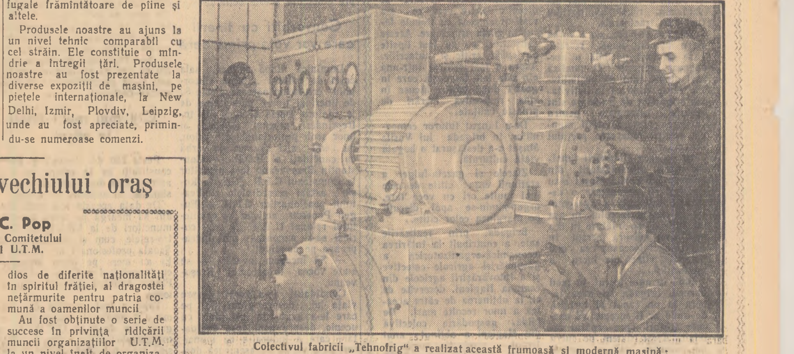
Colectivul fabricii „Tehnofrig” a realizat această frumoasă și modernă mașină: compresorul de amoniac.
