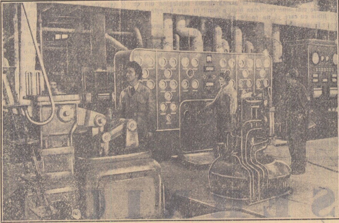
În sala de mașini a centralei electrice de termocifere din Bozești s-a terminat ultima probă pentru punerea ei în funcțiune.
