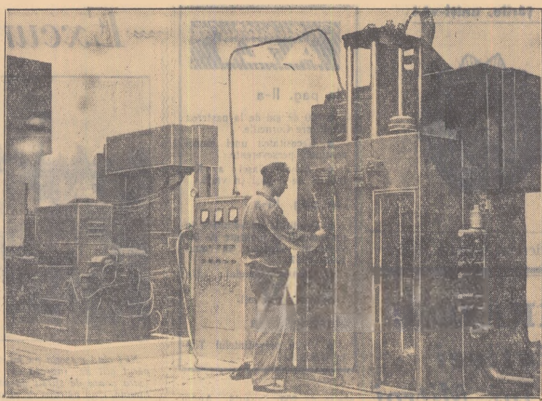
Stația de călire a uzinelor de autocamioane „Steagul Roșu” din Orașul Stalin acționează cu ajutorul curentului de înaltă frecvență. In fotografie: tînărul C. Constantin, unul dintre călătorii fruntași ai uzinei. Foto: AGERPRES
