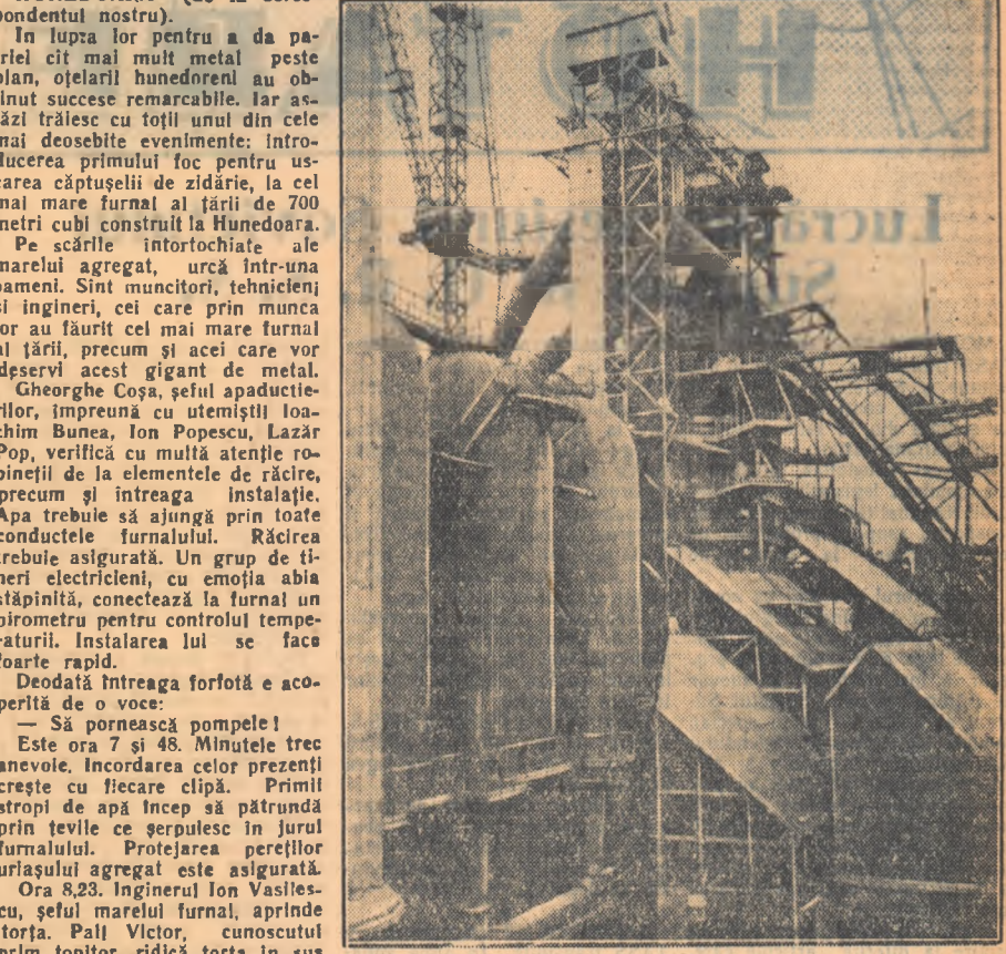
Noul furnal de 700 metri cubi de la Hunedoara
