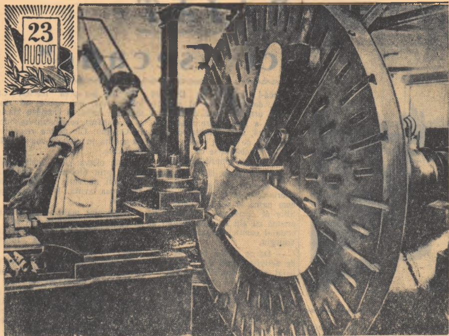
Iată-l pe utemistul Constantin Capotă, unul dintre fruntașii secției de strungărie de la șantierul naval din Galați, lucrând la o elice de tracțiune pentru remorcherul de mare de 1200 c.p. Antrenat în întrecerea în cinstea zilei de 23 August, strungarul Constantin Capotă își depășește norma zilnic în medie cu 37 la sută.
