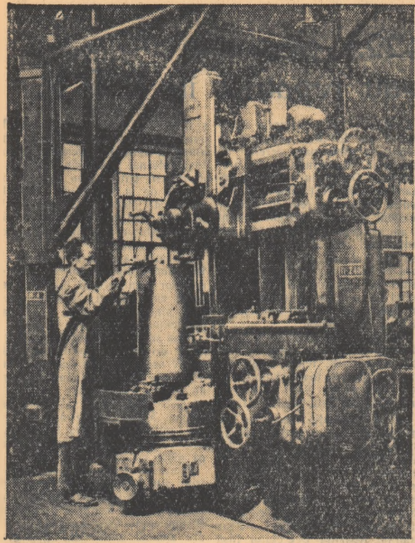
La Fabrica de piese de schimb C.F.R. din Galați lucrează mulți tineri bine calificați, bine pregătiți. În fotografie: lucrător la un ștampilor, un tambur necesar unei benzi rulantă. Datorită unei bune organizări a muncii și a justei folosiri a capacității de lucru a mașinii, el realizează în mod permanent importante depășiri de normă, care în prima decadă a lunii august au atins cifra de 180 la sută.
