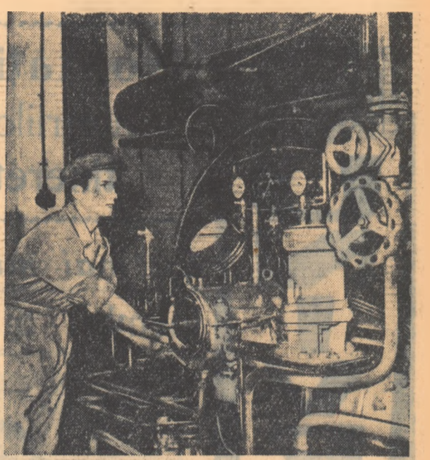
De curînd la rafinăria nr. 8 din Moldova a intrat în funcțiune, cu două luni înainte de termen, o nouă instalație de cracare termică. În fotografie: fochistul Vasile Vărărașu regînd intrarea țijeului în cuptor.
