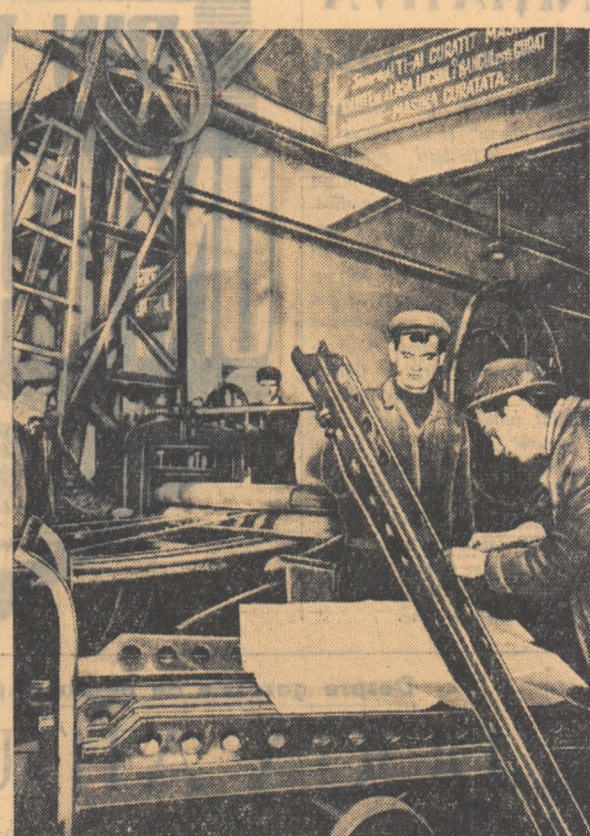
Uzinele „Semănătoarea” din București este una din întreprinderile fruntașe, care lucrează în contul anului 1957. Printre produsele noi pe care le-a realizat anul acesta întreprinderea se află și mașina de recoltat stafii. În fotografie: membrii brigăzii de tineret, condusă de Anghel Dumitru împreună cu controlorul tehnic Aristide Popescu, fac revizuire teșeurilor de la transportorul mașinii de recoltat stafii.
