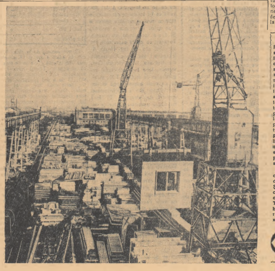
Stimulul de construire a caselor din prefabricate aduce însemnate economii. Șantierul de construcție care folosesc prefabricatele apar ca unități de montaj. Timpul de realizare a unui bloc cu 24 apartamente se reduce de la 5-6 luni la maximum 2 luni.
