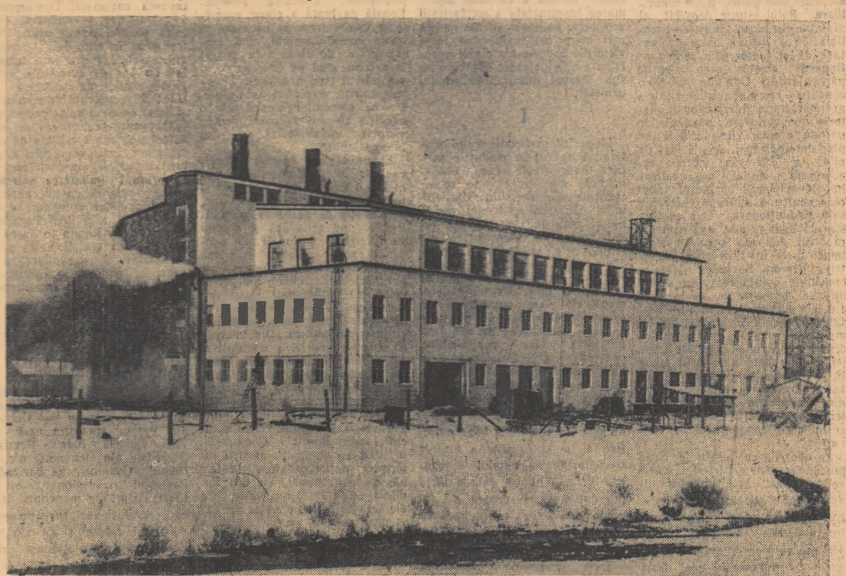
Termocentrala de la Combinatul chimic nr. 1 din regiunea Stalin, es la prima centrală electrică proiectată în întregime în țara noastră. În fotografie: termocentrala de la Combinatul chimic care a intrat de curînd în funcțiune.
