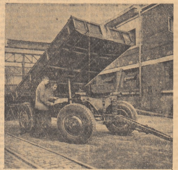
La uzinele „Steaua Roșie” din București a început fabricarea în serie a noului remorcăz basculante mecanizate de 4 tone, care servește la transportul de materiale pe șantierele de construcții și poate fi remorcăz de tractor, avînd descărcarea laterală și pe spate.
