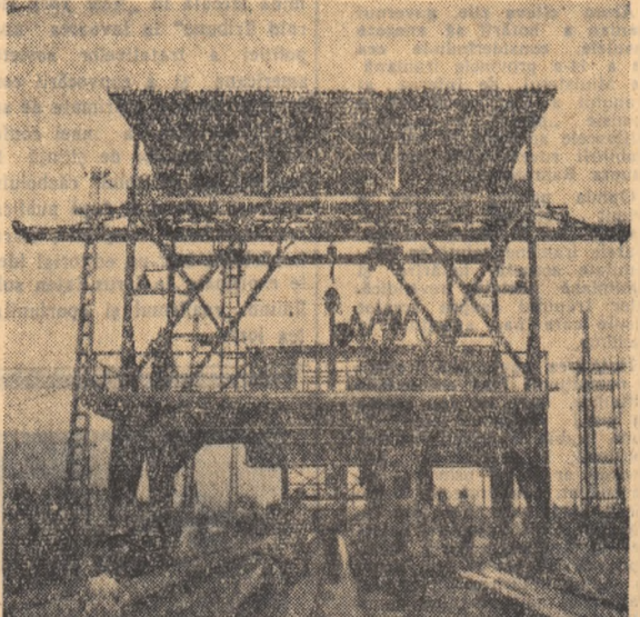
De curînd a intrat în funcțiune la fabrica de prefabricate din Capitală o nouă instalație „Stasa” sosită din R.D. Germană. Instalația servește la turnarea planșelor de beton armat prefabricate toate operațiile executîndu-se mecanizat. Noua instalație poate produce anual produse prefabricate pentru 2.000—3.000 apartamente cu 3 camere și anexe, este deservită de 10 oameni pe schimb și înlocuiește munca a 150 oameni. În fotografie: Vedere generală a noului instalații „Stasa” de turnare a planșelor prefabricate.
