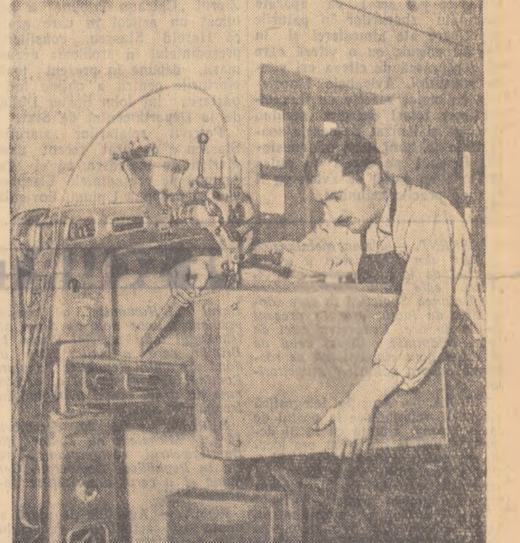
La întreprinderea „Stăruința” din Capitală a intrat în funcție, în fața experimentală, o nouă secție de bunuri de larg consum din poliorură de vînt.
