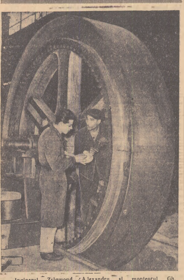
Inginerul Zsigmond A. Alexandru și monteurul Gh. Stănicuț de la uzina „23 August” din Capitală, controlînd fixarea celor două jumătăți de volant, plesă ce urmează să fie montată la compresorul de amoniac
