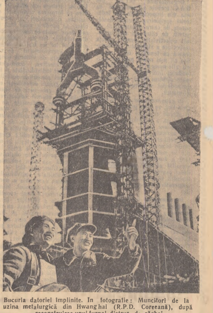
Bucuria datoriei împlinite. În fotografie: Muncitorii de la uzina metalurgică din Hwang hai (R.P.D. Coreeană), după reconstruirea unui furnal distrus de război.
