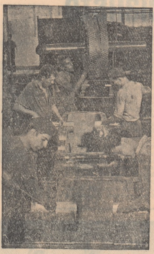
Uzinele Mao Tze-dun, secția mecanică ușoară. Dumitru Pană împreună cu membrii din brigada sa lucrează la operațiile de rețușare la reductorul pentru utilaj petrolifer
