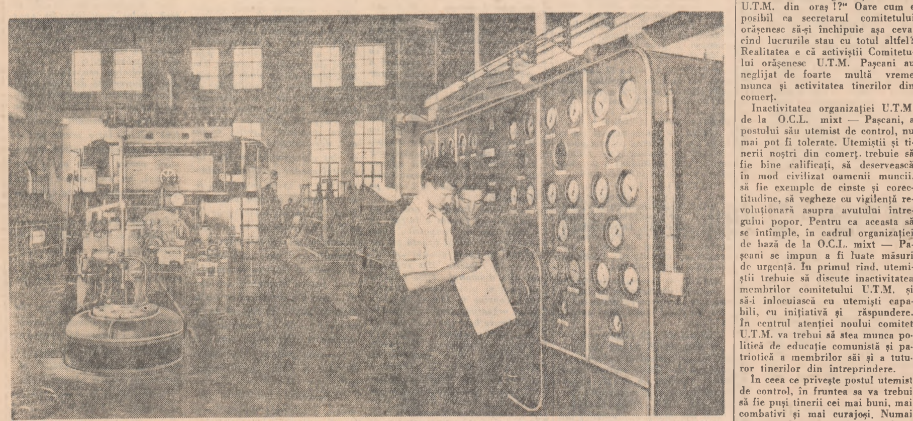
La termocentrala de la Borzești a început montarea celui de-al treilea turbo-generator de 25 M.W. și cazanul de înaltă presiune. În cursul anului viitor termocentrala de la Borzești își va mări puterea instalată de la 100 M.W. la 225 M.W. Montajul primului turbo-generator de 50 M.W. va începe la începutul anului viitor. În fotografie: Șeful de tură E. Toader și mecanicul de turbină M. Antohie în timpul lucrului; jînera preslunii constante.
