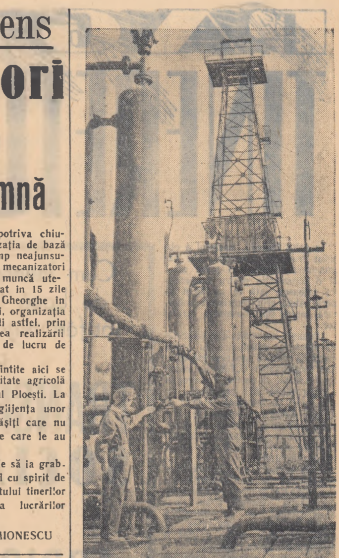
Brigadierul șef Mihal Dobre de la șchea petrolieră Boldești explică elevului Vasile Romulus modul de funcționare a unui parc de separatoare.
