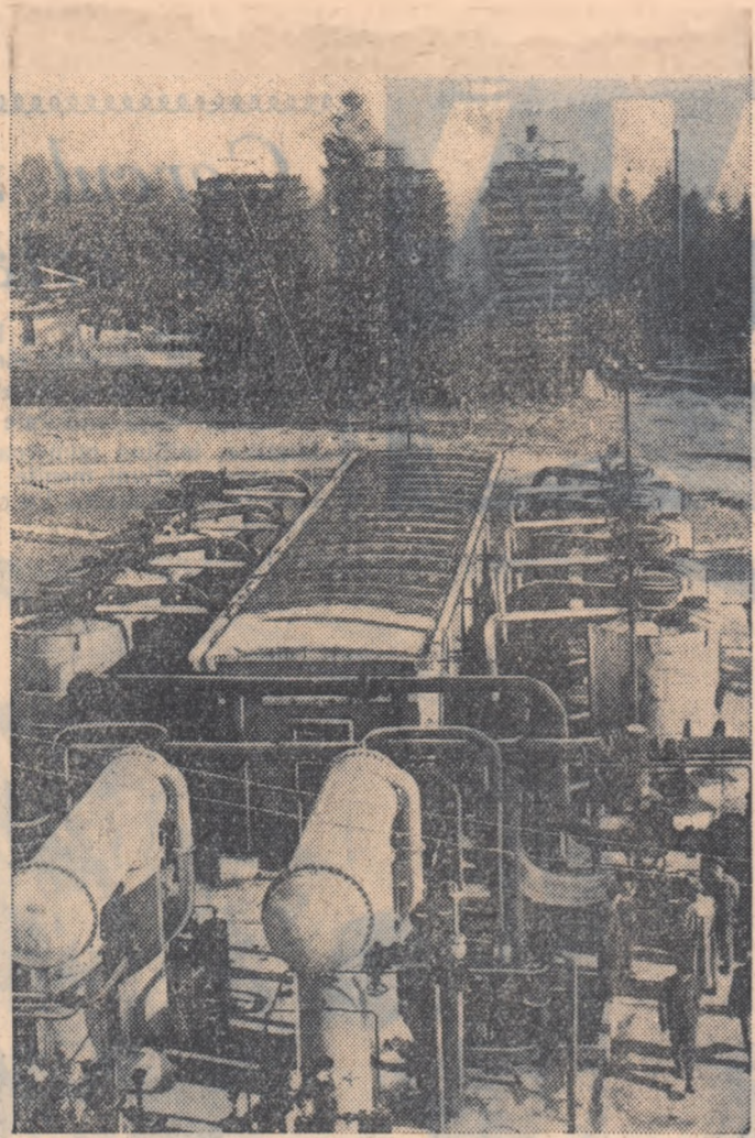
Stația de dezbenzinare de la Modrîșu, regiunea Bacău
