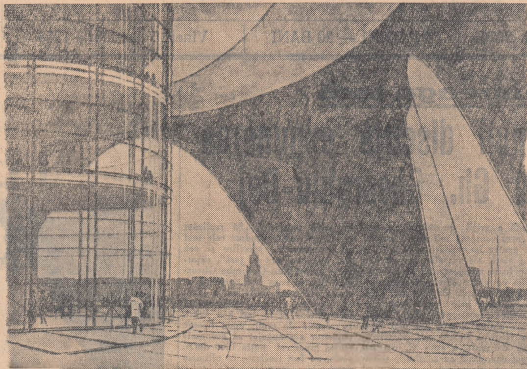
În cursul anului viitor va începe la Moscova construcția noului turn de televiziune din beton armat monolit. Înălțimea lui va fi de 508 metri. Diametrul bazei va fi de 65 metri, iar cel al vîrfului de 7 metri. În fotografie: Vestibulul părții inferioare a turnului.
