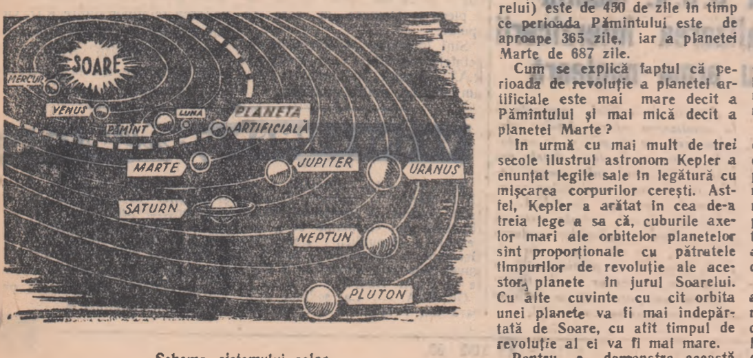
Schema sistemului solar
