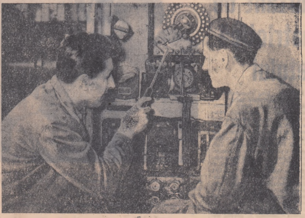
Impreună cu comunistul Al. Tudorache, utemistul Vasile Marin de la uzinele „Republica” a realizat un dispozitiv automat pentru comanda mașinii de deșoțat. Cu ajutorul acestui dispozitiv se realizează o turație mai mare a mașinii ceea ce duce la creșterea productivității muncii. În fotografie cei doi muncitori urmărend funcționarea dispozitivului. Foto: N. STELORIAN
