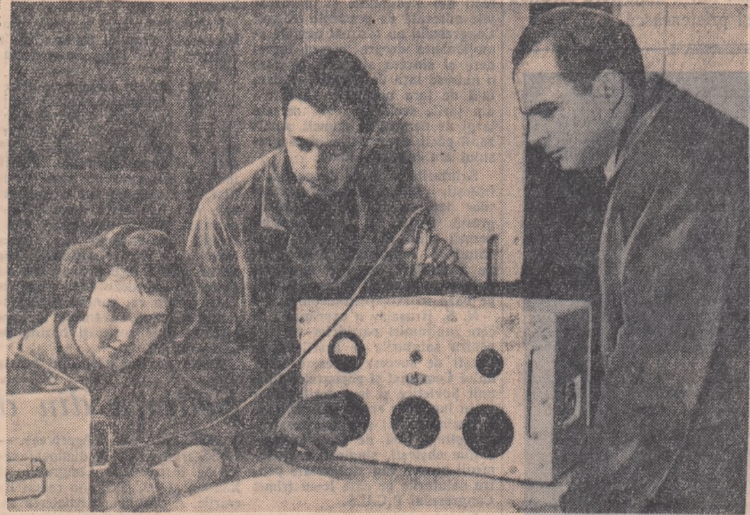
Colectivul de tehnicieni al întreprinderii „Electrotehnica” din Capitală a realizat un nou produs-aparat de electrochirurgie și electrocoagulare cu o putere de 200 Wați. Noul produs a fost experimentat cu succes în clinicele de chirurgie din Capitală. În fotografie: ing. Stoiculescu Ștefan, proiectantul noului aparat, ing. Florica Ștefănescu și Ștefan Frinculescu măsurînd în laborator caracteristicile noului aparat. Foto: AGERPRES
