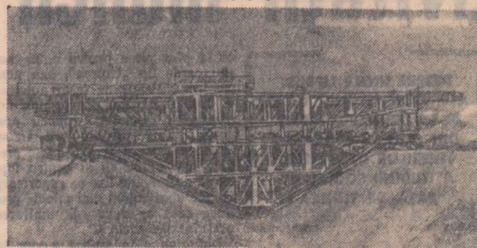
Cu ajutorul mașinii sovietice de mai sus se poate asferta beton într-un strat gros de 30 cm. pe suprafață pînă la 1500 mp. Lungimea mașinii este de 42 m, iar înălțimea egală cu cea a unei case cu 4 etaje. Agregatul deservit de doi oameni înlocuiește munca a 250 muncitori.
