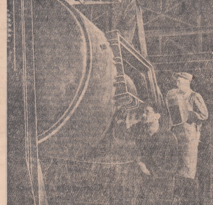
Utemistii Ion Bărbieru și Ion Irla da la Uzinele „Șteaur-Roșie” lucrind la montarea autoclavelor de 750 litri pentru industria alimentară. Aceste autoclave se fabrică pentru prima oară in uzină.
