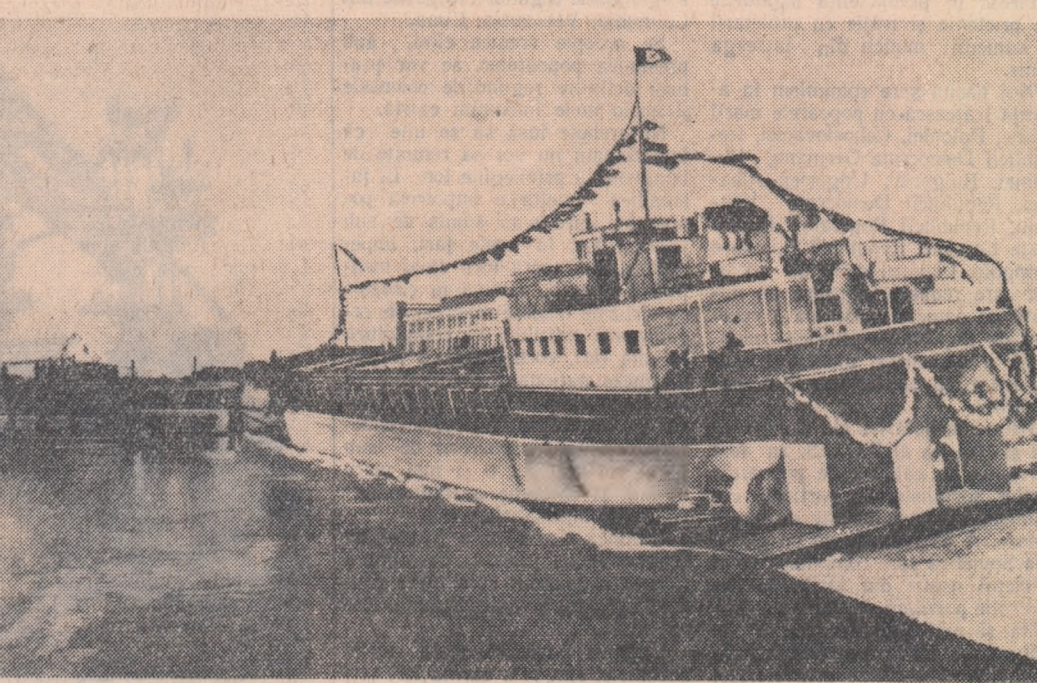
În ziua de 19 aprilie la Șantierul naval Oltenița a fost lansată la apă o motonavă cu o capacitate de 2.000 tone. Motonava a fost lansată cu 4 luni înainte de termen în cinstea zilei de 1 Mai. Ea este destinată pentru transporturile de mărfuri pe fluvii și lacuri de acumulare și este înțărîtă pentru navigația pe șoari. Are două motoare de 500 G.P., fiecare cu o viteză de 18 km. pe oră.
