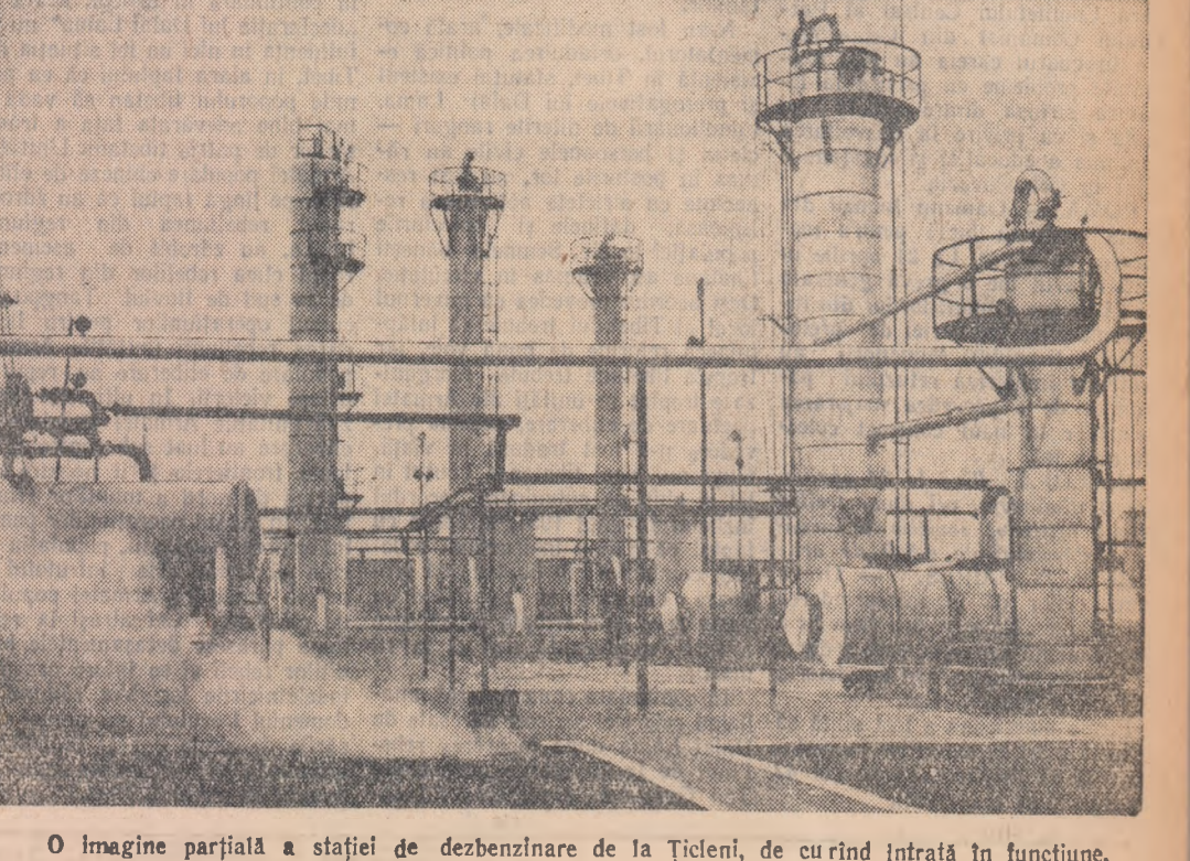
O imagine parțială a stației de dezbenzinare de la Tîcieni, de curînd intrată în funcțiune.
