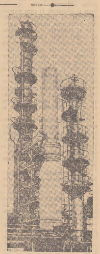
O parte din instalația de absorbție și fracționare a gazelor de la o rafinărie de la Onestî.
