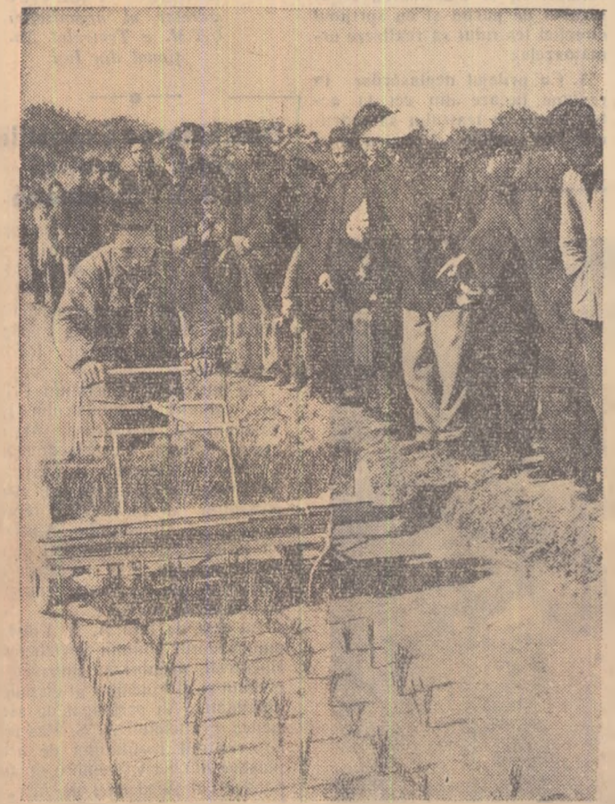
Institutul de cercetări agro-tehnice din provincia Guansi (R.P. Chineză) a creat un nou tip de plantator de orez care ridică productivitatea muncii de șase ori față de plantarea orezului cu mâna. Experiențele au arătat că mașina corespunde condițiilor soluției din regiunea Guansi — unul din marile centre ale culturilor de orez din R.P. Chineză. În fotografie: Aspect în timpul unei experiențe cu noul tip de plantator.
